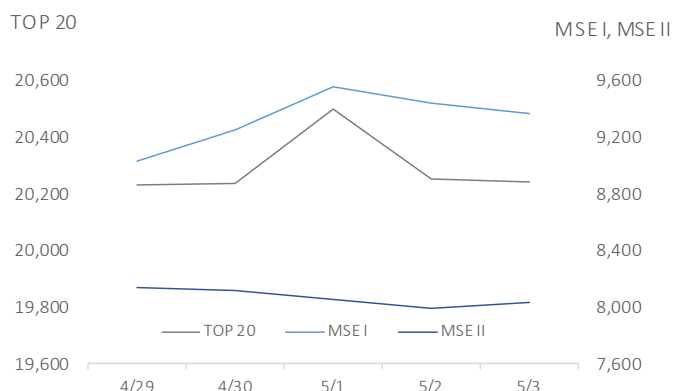
MSE Индекс
